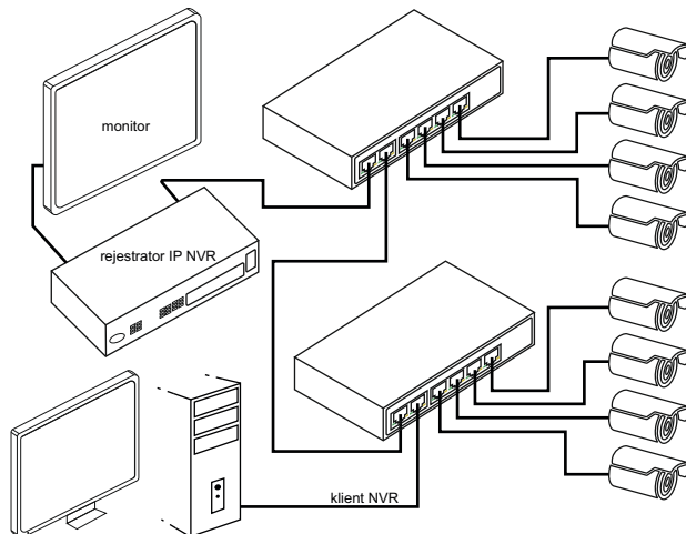
Schemat rozbudowy systemu kamer IP CCTV
